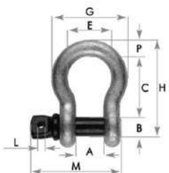
Chei tachelaj omega de înaltă rezistență cod a-052-xx
