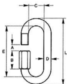
Carabine rapide cod a-064-xx
