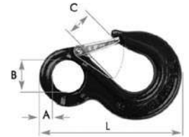
Cârlige de ridicare cu inel și siguranță oțel C40, cod a-104-xx
