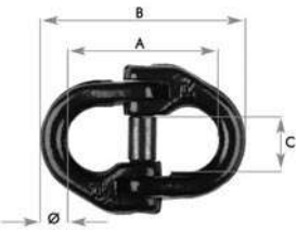
Chei tachelaj drepte de înaltă rezistență cod a-051-xx
