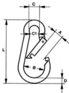
Carabine zincate cu dîchet cod a-068-xx
