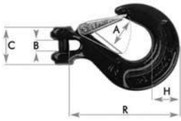
Cârlige de ridicare Clevis cu siguranță cod a-510
