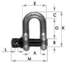
Chei tachelaj drepte de înaltă rezistență cod a-051-xx
