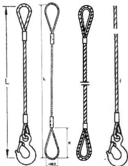
Sufe de cablu cu un braț, prevăzute cu ocheti sau cu accesorii diverse la capete
